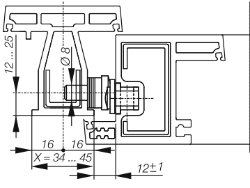
Sonderfall: Höhenchnitt KSP EBZ 16mm am Kunststoff-Fenster
